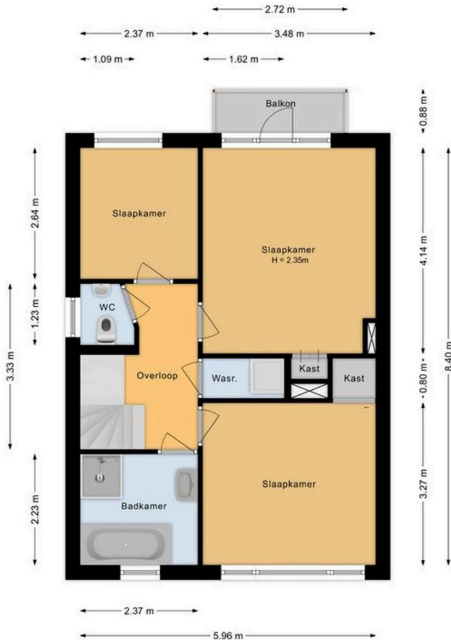
Golfbaan 6 Noordwijk 1e Verdieping
